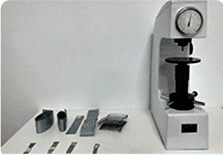
Prueba de Dureza
